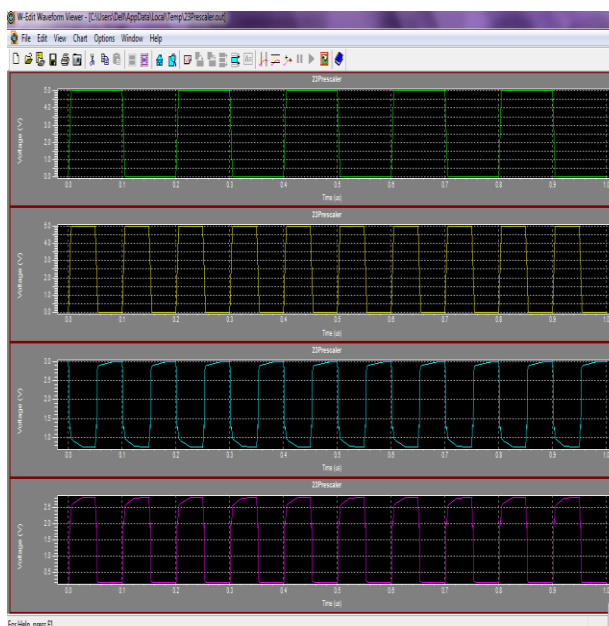
Fig 8: DFF1 Output Waveform
